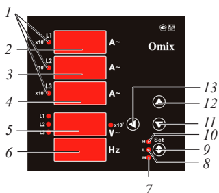
Рис. 1 – Управляющие элементы
