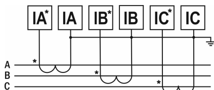
Рис. 8 – Подключение трансформатора тока x/5 А
