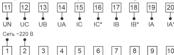
Рис. 4 – Клеммы подключения
