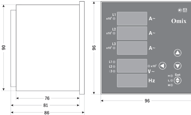
Рис. 3 – Размеры прибора
